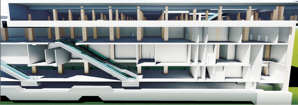
地铁1号线太原站东广场车站断面效果图
