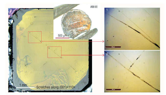
用AM-III刻划金刚石(001)面留下的划痕(资料照片)。8月14日，记者从国家重点实验室之一的燕山大学亚稳材料制备技术与科学实验装置获悉，新型非晶材料(AM-III)近日在该实验室成功合成。
