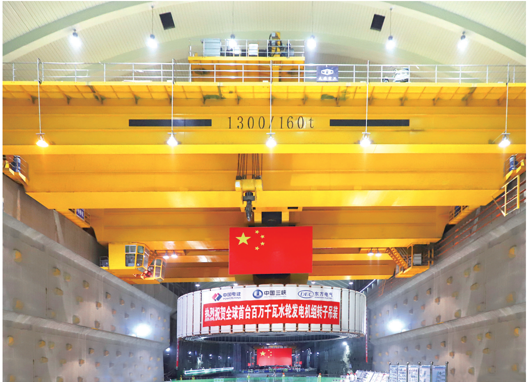
太重集团研制的世界上最大的1300吨桥式起重机
