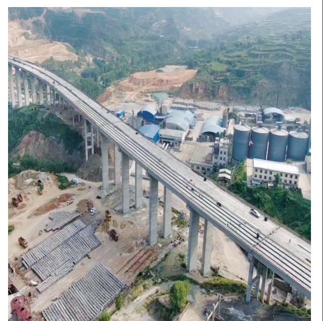
太原西北二环高速公路阴家沟特大桥T梁架设已全部完成。
