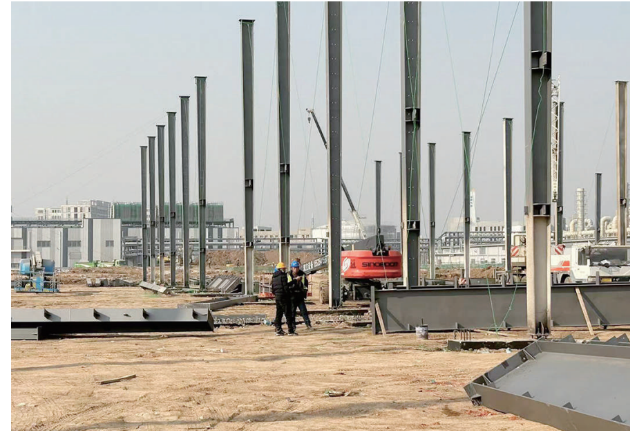
作业人员指挥直臂式高空吊装车将一根根加工好的钢柱安装到顶。
