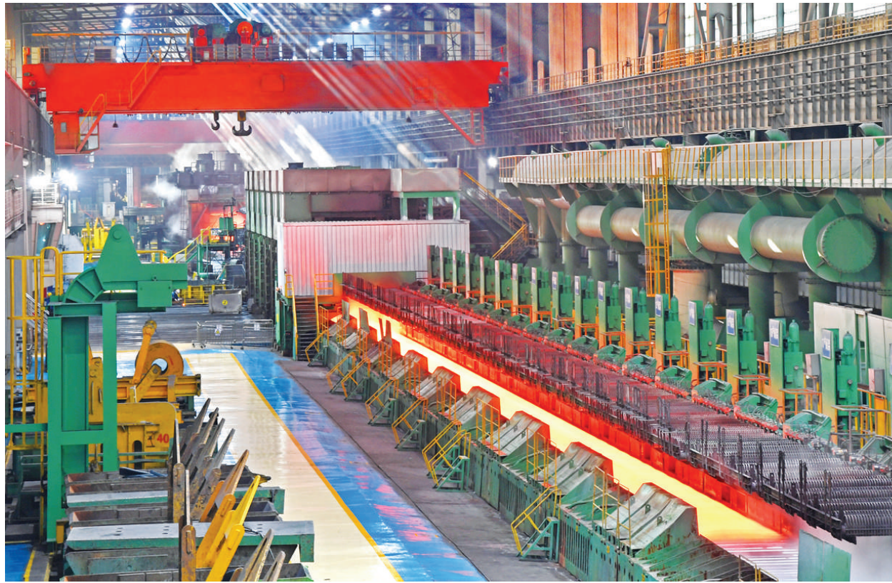
1月6日，中国宝武太钢集团热连轧2250mm生产线在轧制超厚规格热轧卷板。日前，太钢通过技术创新，首次轧制成功31毫米超厚规格高强度建筑用热轧卷板，达到行业同规格轧制厚度先进水平，成为目前国内唯一能够生产31毫米超厚规格热轧卷板的企业，具备了超厚规格卷板供货能力。王旭宏 摄
