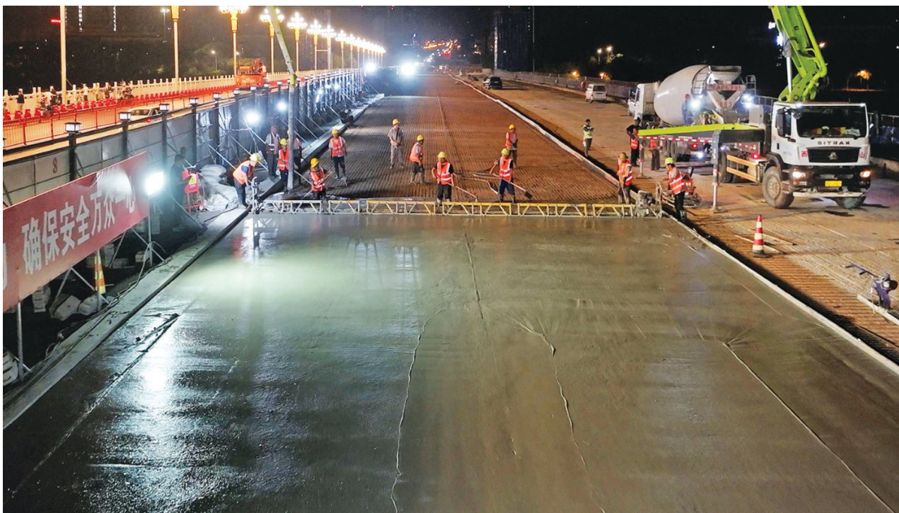
8月11日凌晨，市政建管中心市政桥梁管理所施工人员在迎泽大桥北半幅桥面进行混凝土浇筑。自7月21日迎泽大桥北半幅桥面开始维修加固施工以来，建设人员克服高温天气和降雨影响昼夜奋战，目前工程进展顺利。
