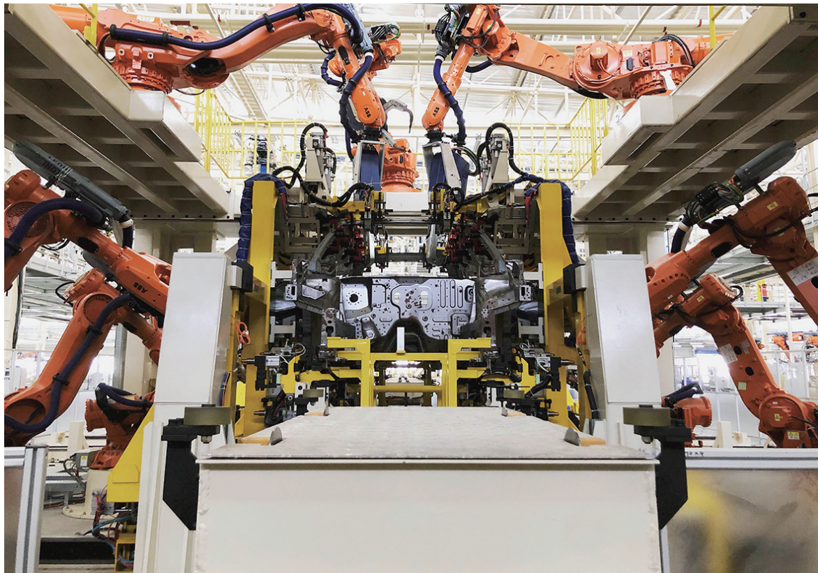
广州明珞装备股份有限公司的海外项目生产线(2019年4月10日摄)。新华社 发
