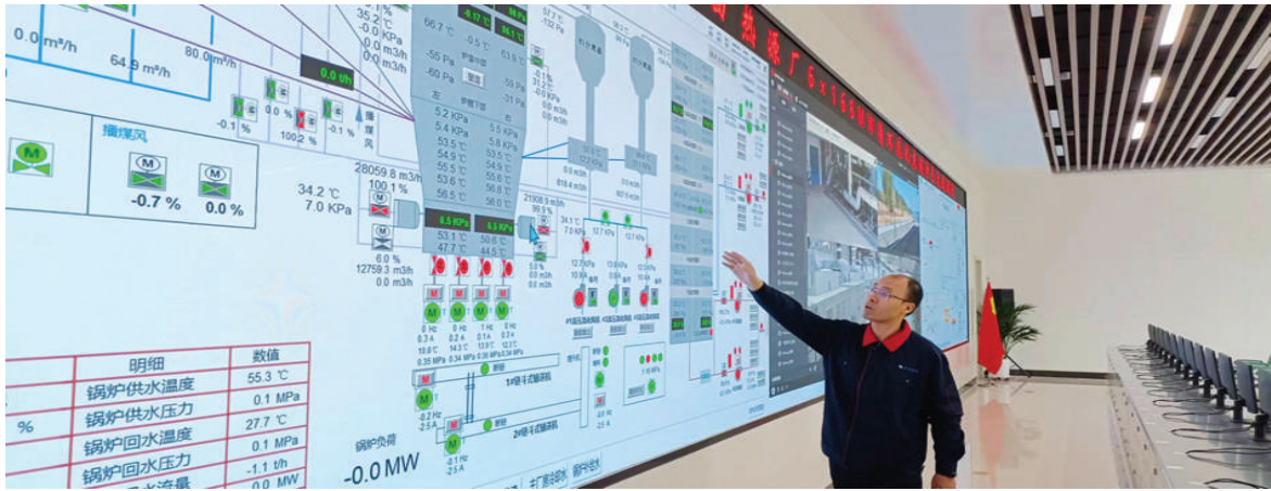
阳曲热源厂点炉投产以来运转良好。图为技术人员正在观测锅炉压力表、流量表。
